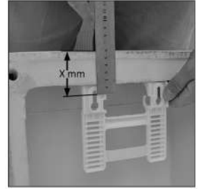
6 Rezervuar klozetin üzerinden alınarak şekilde görüldüğü gibi rezervuarın üst noktası ile Braketin montaj deliği arasının ölçüsü (x mm) alınır.
