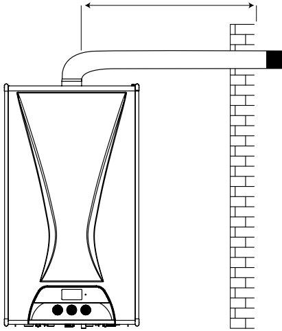
a) Tek 90° dirsekli örnek baca tesisi
