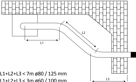
c) Tek 90° ve 45° dirsekli örnek baca tesisi
