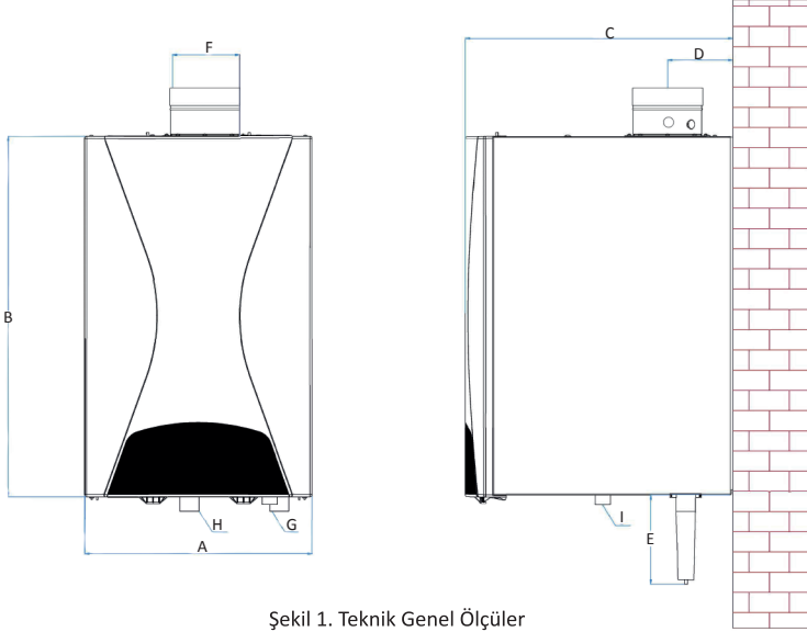
Şekil 1. Teknik Genel Ölçüler
